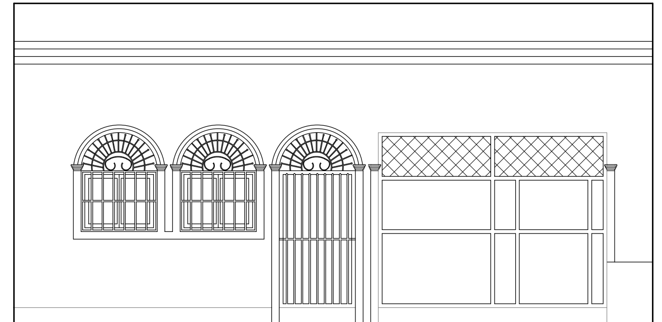
EDIFICAÇÃO RC-184 FACHADA LATERAL ESC. _____ 1/50
