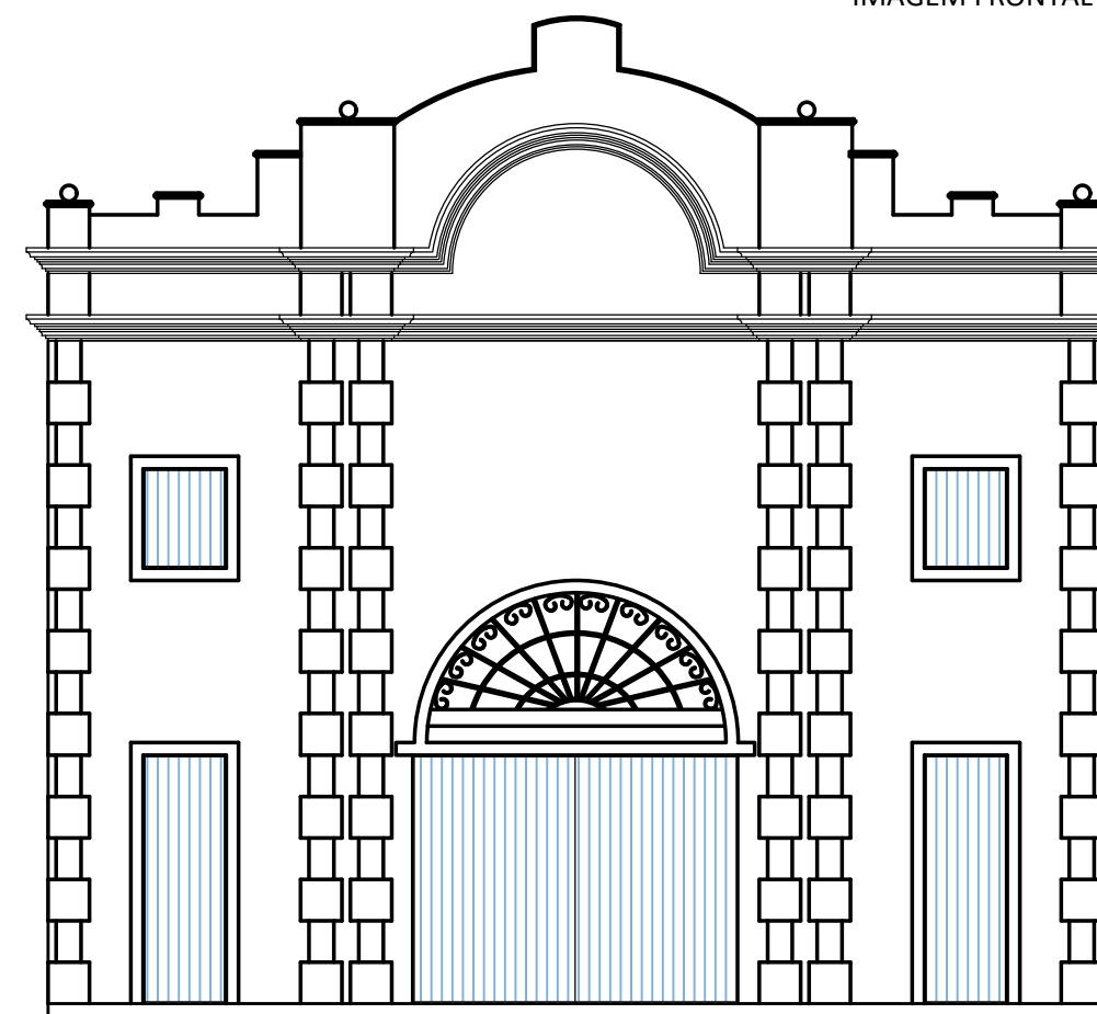
EDIFICAÇÃO RC-33 FACHADA FRONTAL ESC. 1/100
